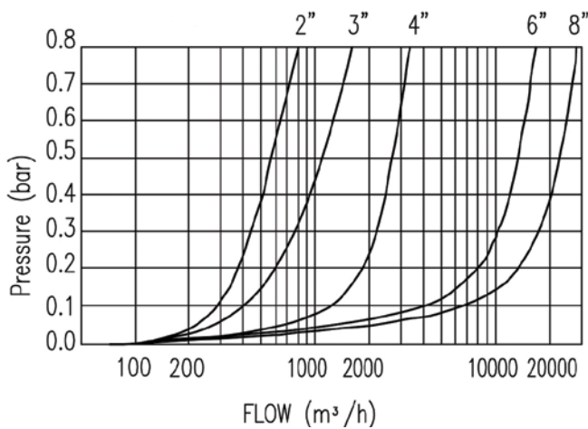
Outflow / Отток / Odpowietrzanie
